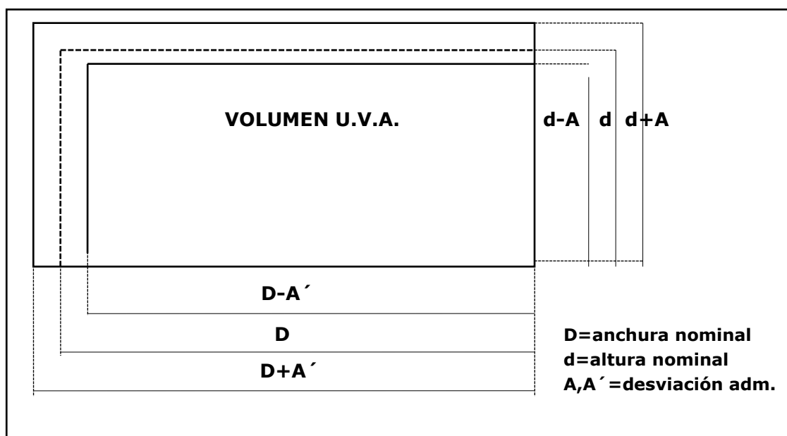
Figura E.5 Tolerancia de Angularidad
